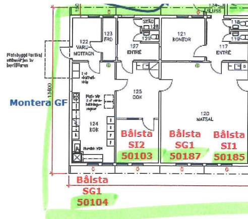
PLAN, SKALA 1:100
