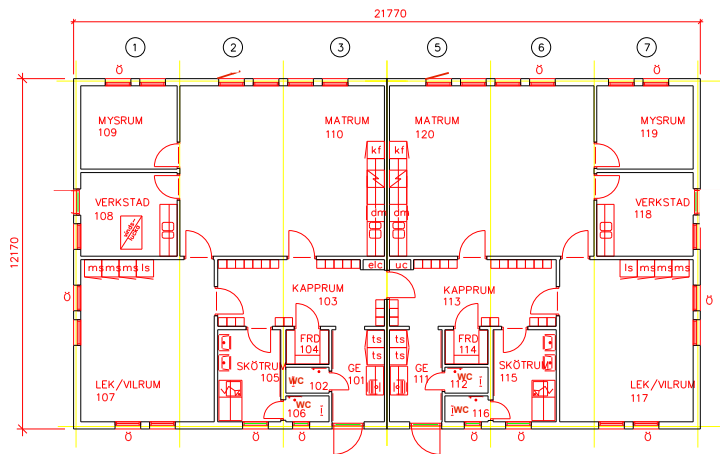
PLAN BYA-265 m 2
