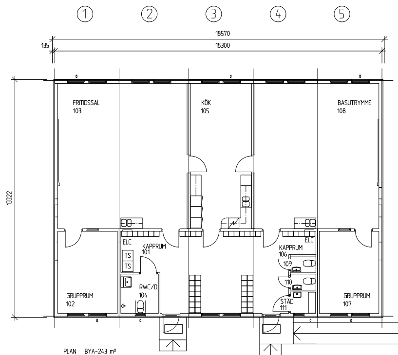
PLAN BYA-243 m 2
