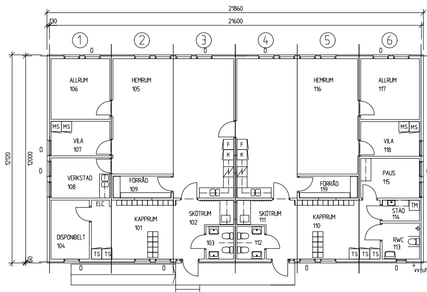
PLAN BYA- 265 m 2
